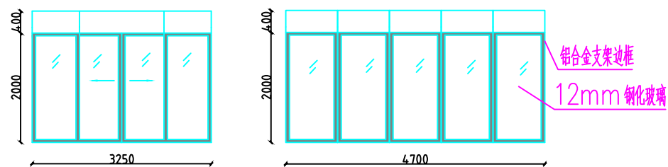
门诊四楼中医科安装玻璃隔断立面图
