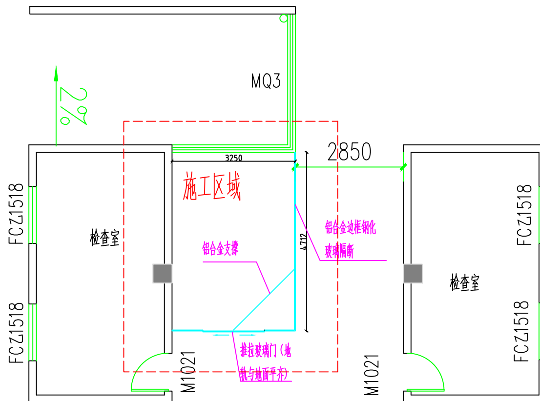
门诊四楼中医科安装玻璃隔断平面图
