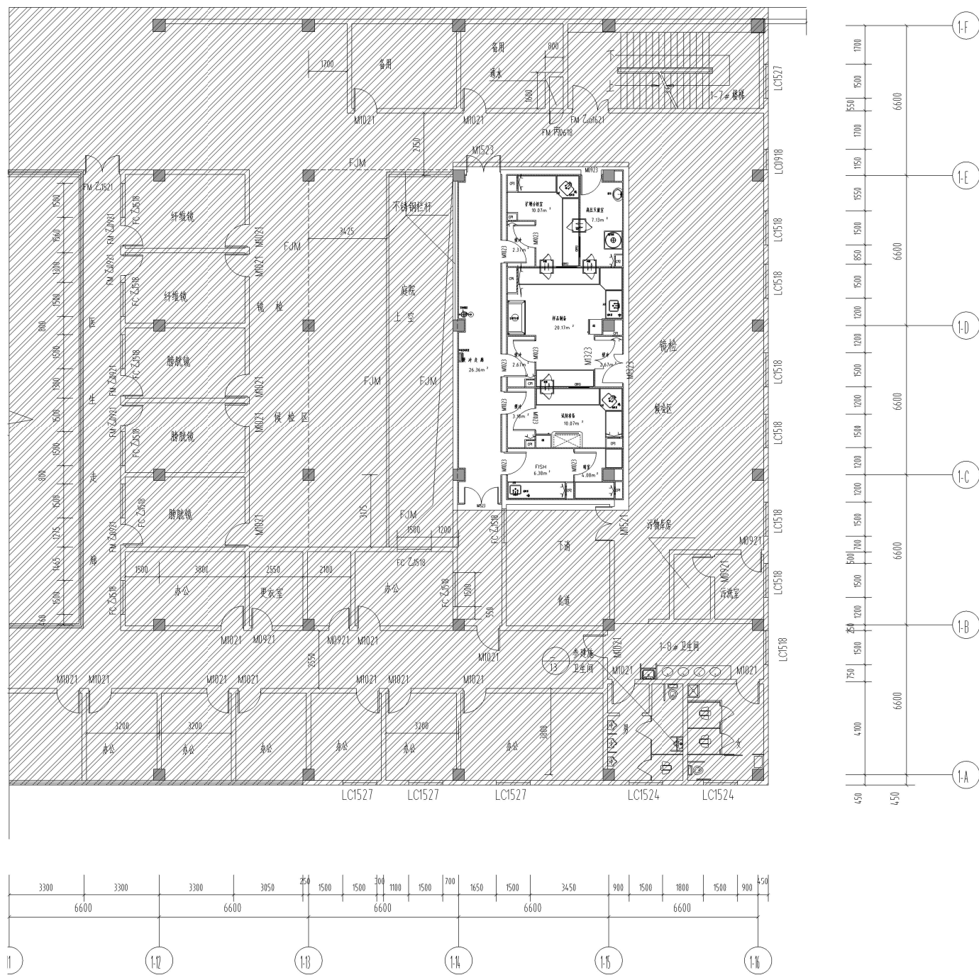
三层分子实验室平面图 1:100
